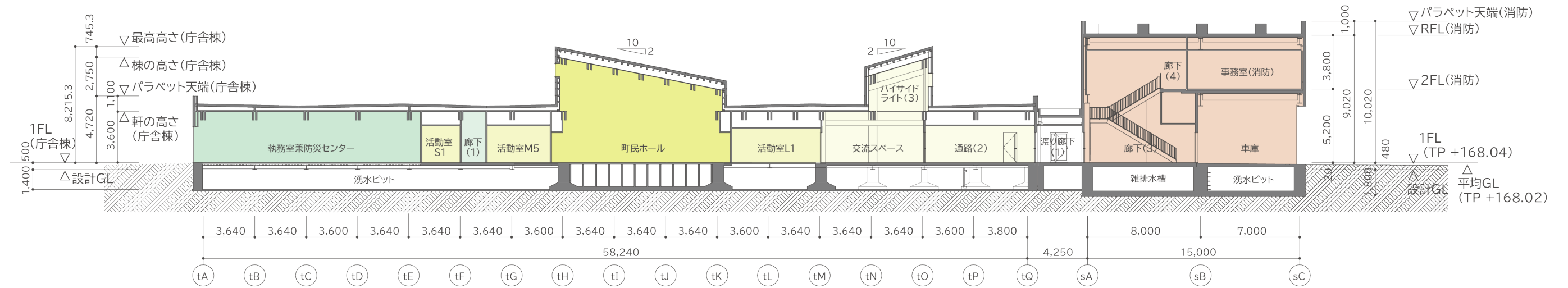
Y1断面図
