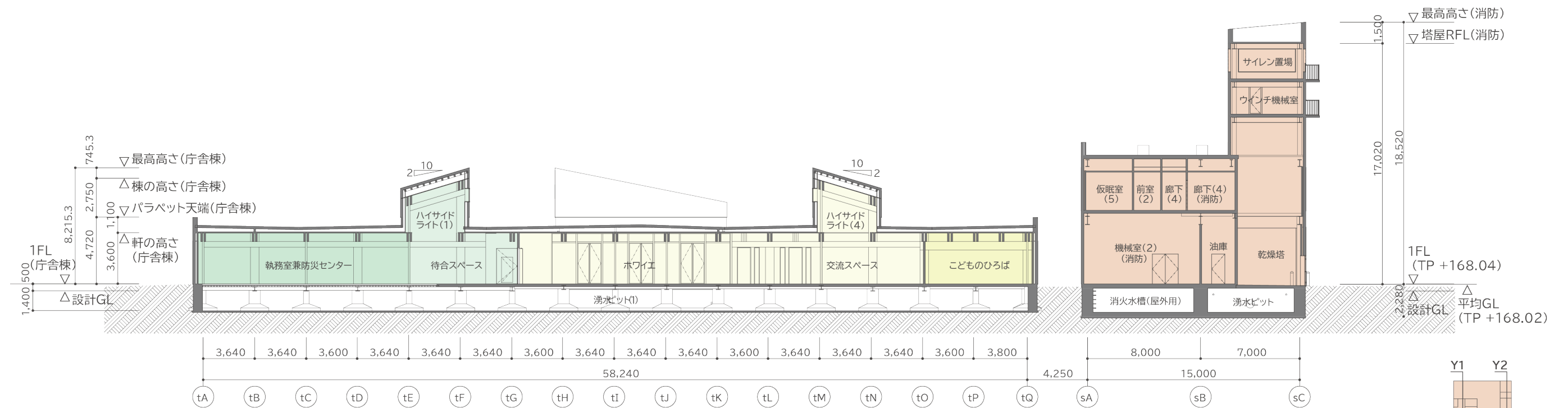
Y2断面図
