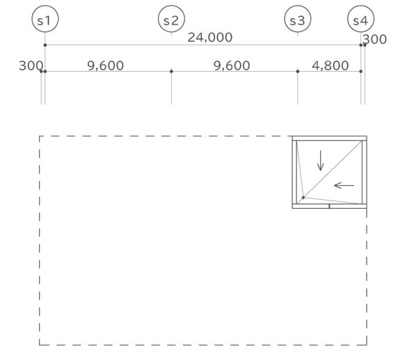
塔屋屋根伏図
