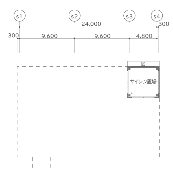
2塔屋階平面図
