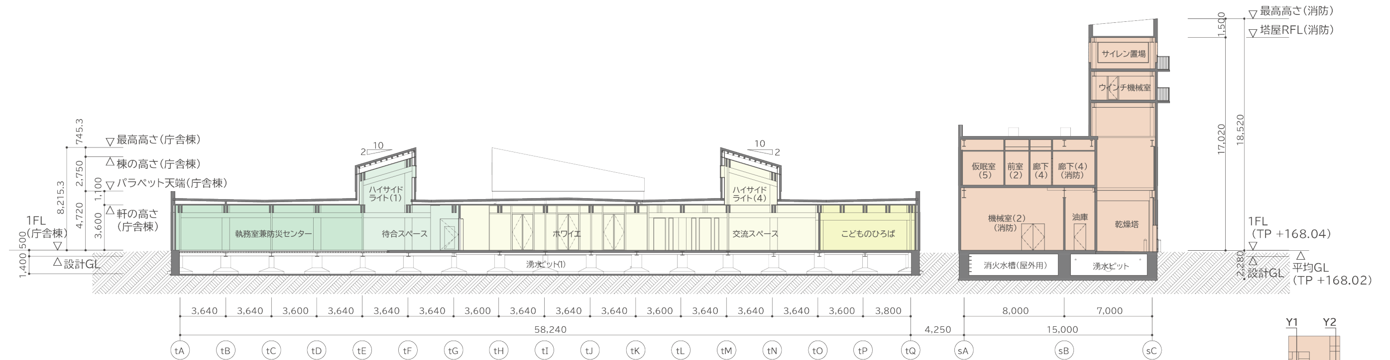
Y2断面図
