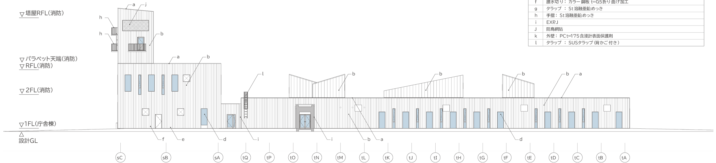
西立面図
