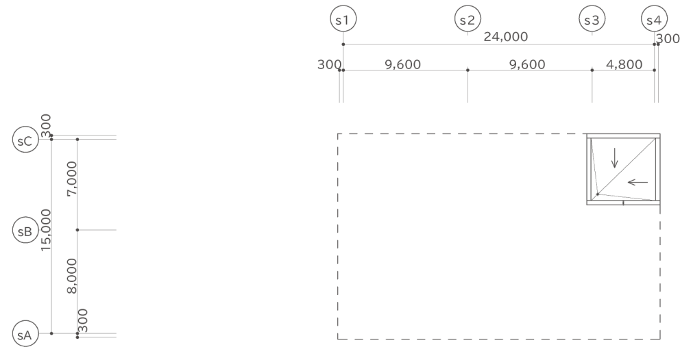
塔屋屋根伏図
