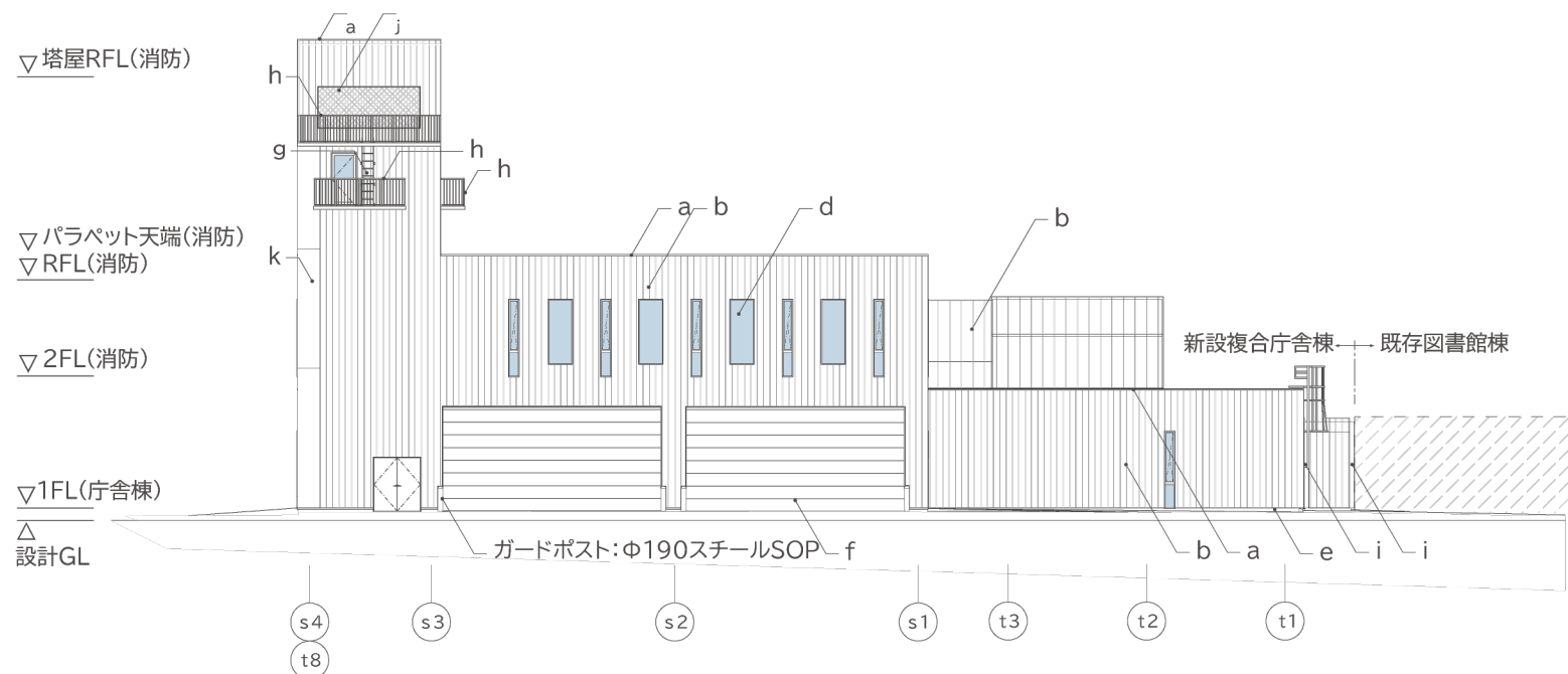
北立面図
