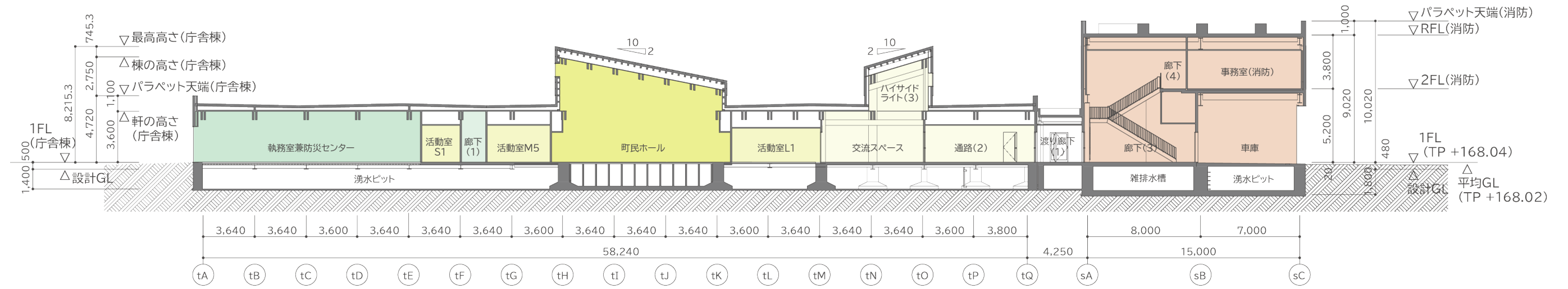
Y1断面図
