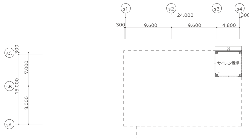
2塔屋階平面図
